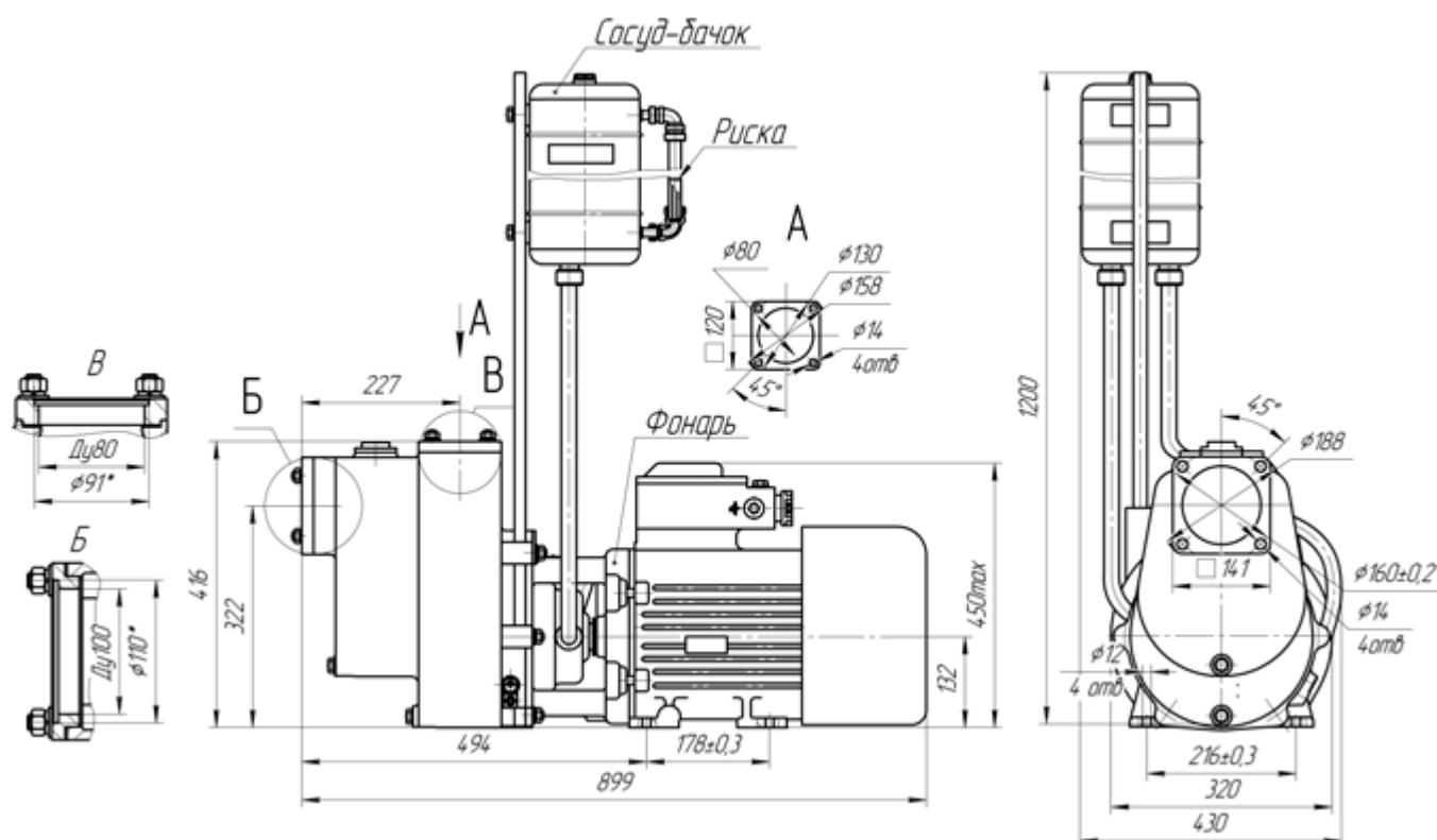
Рисунок Б.12 - Габаритные и присоединительные размеры электронасоса КМС 100-80-180-Е
