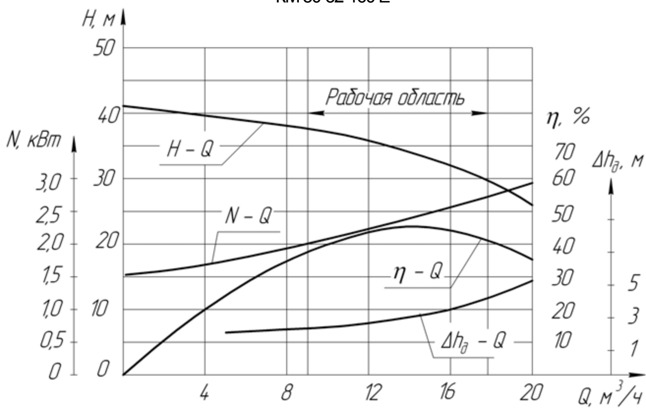
КМ 50-32-160 Е
