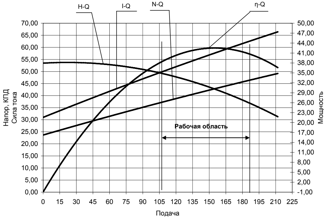
К 125-80-200Е
