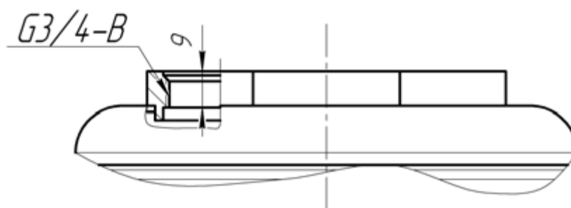
Рисунок Б.16 – Присоединительные размеры под установку датчиков уровня Примечание – Место расположения: крышка сосуд-бачка (2 места) (рисунки Б.6, Б.8, Б.11)
