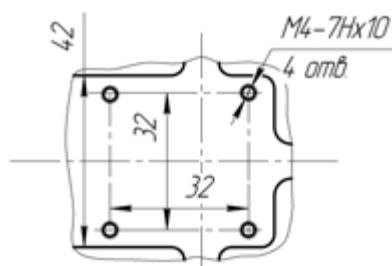
Рисунок Б.13 – Присоединительные размеры под установку датчика вибрации
