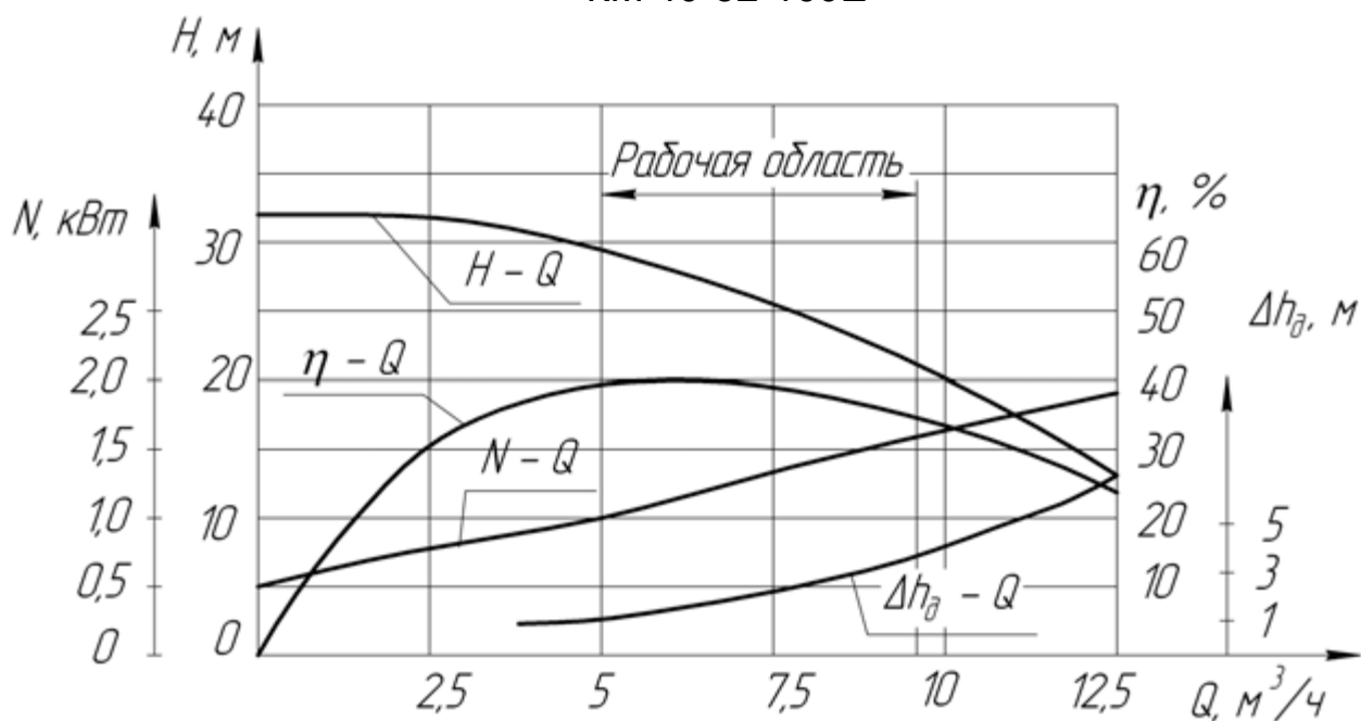
КМ 40-32-160Е
