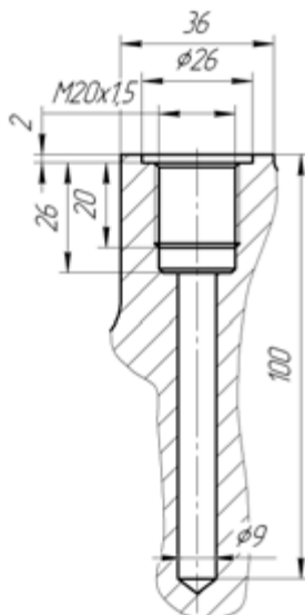
Рисунок Б.15 – Присоединительные размеры под установку датчика температуры (для электронасосов типа КМ, КМС с двойным торцовым уплотнением) Примечание – Место расположения: фонарь электродвигателя насоса (рисунок Б.6, Б.11)
