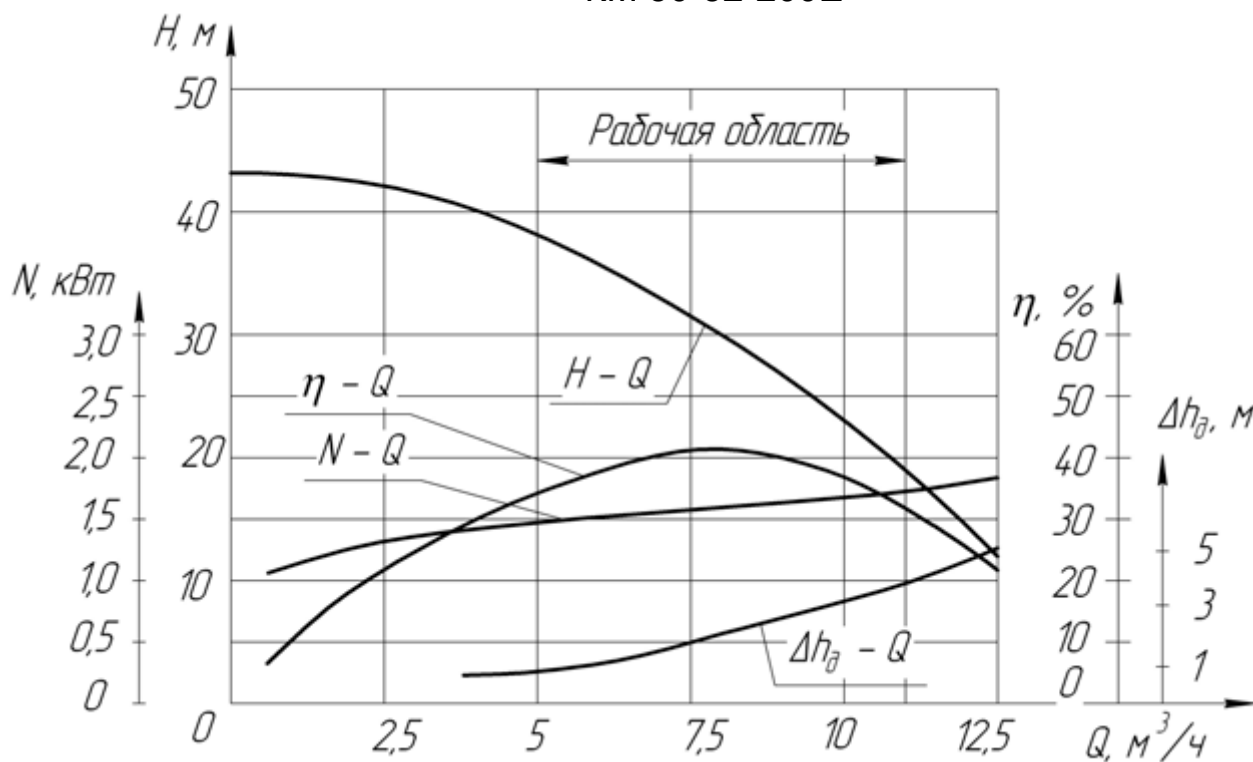
КМ 50-32-200Е
