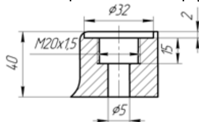
Рисунок Б.14 – Присоединительные размеры под установку датчиков температуры (для агрегатов типа К)
