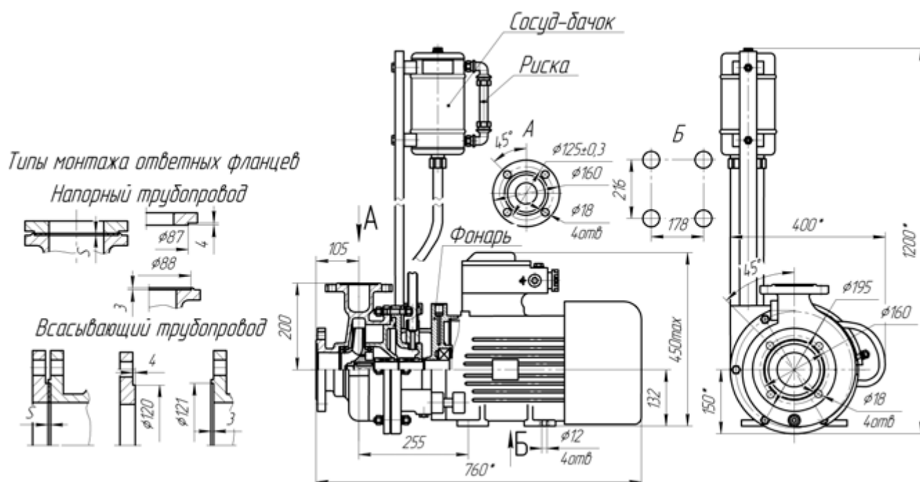
Рисунок Б.7 - Габаритные и присоединительные размеры КМ 80-50-200Е (а,б) с двойным торцовым уплотнением
