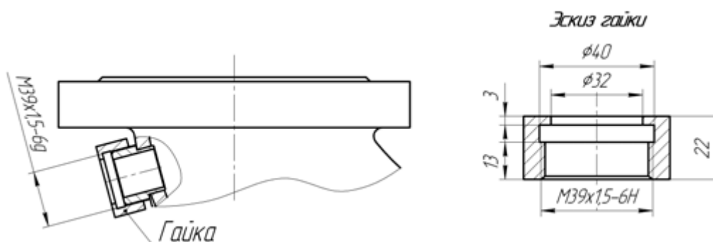
Рисунок Б.17 – Присоединительные размеры под установку датчика «сухого хода» для агрегатов электронасосных К 125-80-200Е, К 200-125-250Е.. Примечание – Место расположения: выходной (напорный) патрубок корпуса насоса (рисунок Б.11)
