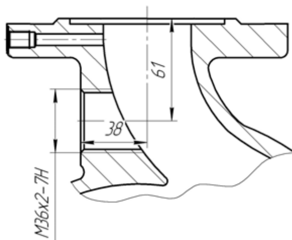
Рисунок Б.9 – Присоединительные размеры под датчик «сухого хода» для электронасоса КМ 80-50-200Е (а, б) с двойным торцовым уплотнением Примечание – Место расположения: выходной патрубок корпуса электронасоса (рисунок Б.7).
