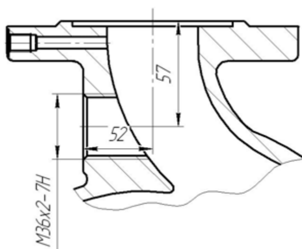
Рисунок Б.10 – Присоединительные размеры под датчик «сухого хода» для электронасоса КМ 100-80-170Е-м, КМ 100-80-160Е-м с двойным торцовым уплотнением Примечание – Место расположения: выходной патрубок корпуса электронасоса (рисунок Б.8).
